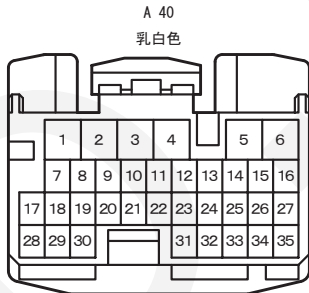
90980-12146 025-29, 040 III-6 025-29, 040 IV-6
