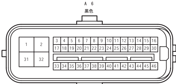
90980-12297 025-42, 187-4
