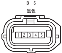
90980-12292 025-5
