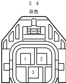
90980-12496 187-3
