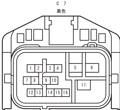
90980-12518 040 III-13, 187-3
