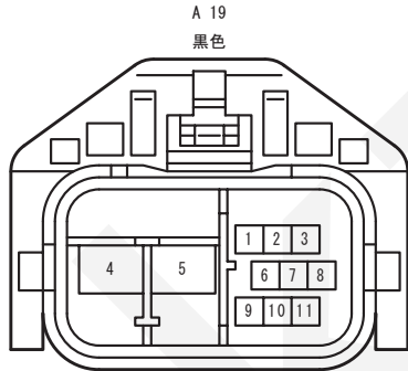
90980-12483 040 III-9, 312-2
