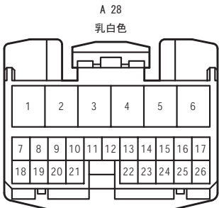
90980-12150 025-20, 090 II-6
