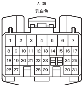
90980-12142 025-24, 040 III-7 025-24, 040 IV-7
