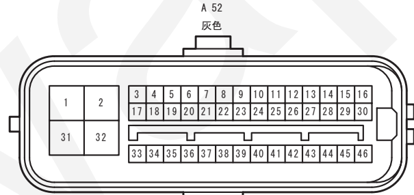
90980-12426 025-36, 187-4
